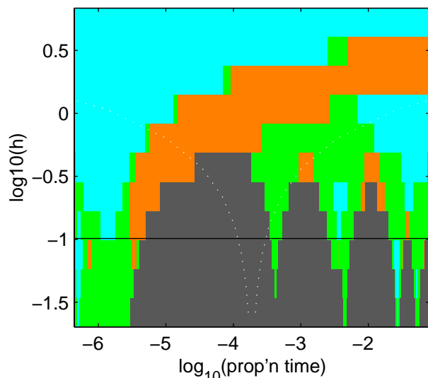
SiCon Map
