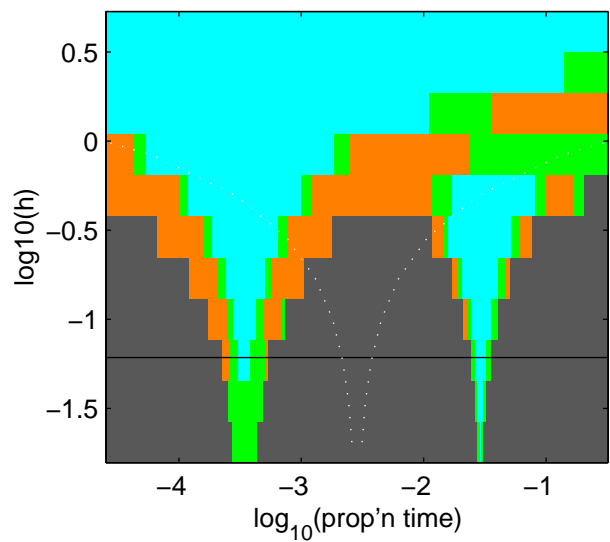
SiCon Map
