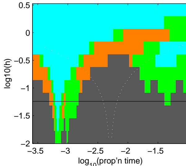
SiCon Map
