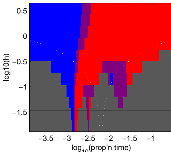
SiCon Map
