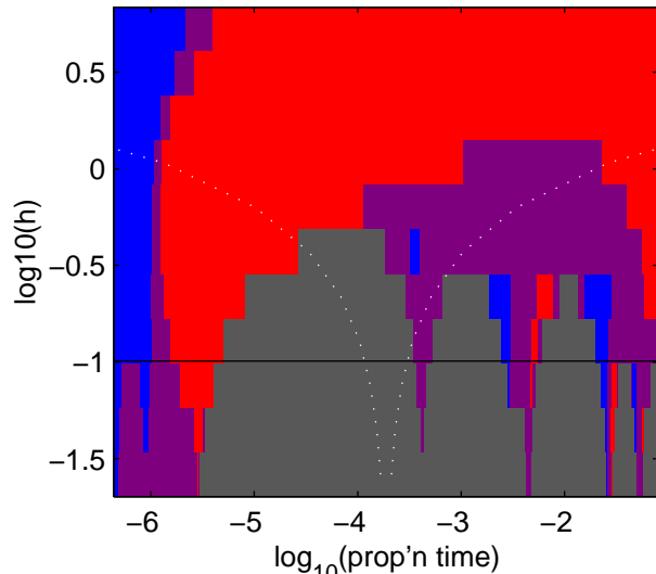
SiCon Map
