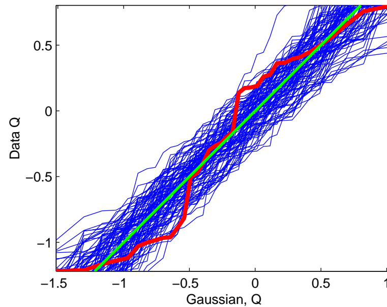
npc = 7 IC 2 Proj's, QQ
