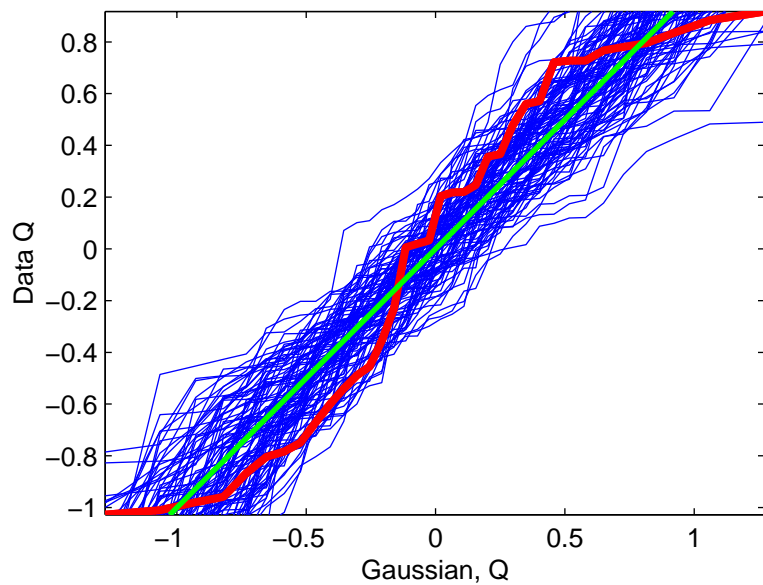
npc = 7 IC 1 Proj's, QQ
