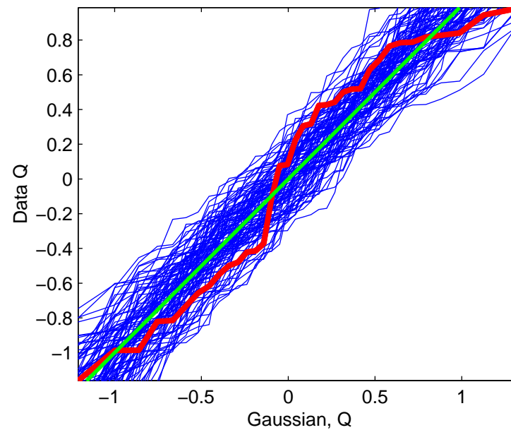
npc = 7 IC 4 Proj's, QQ
