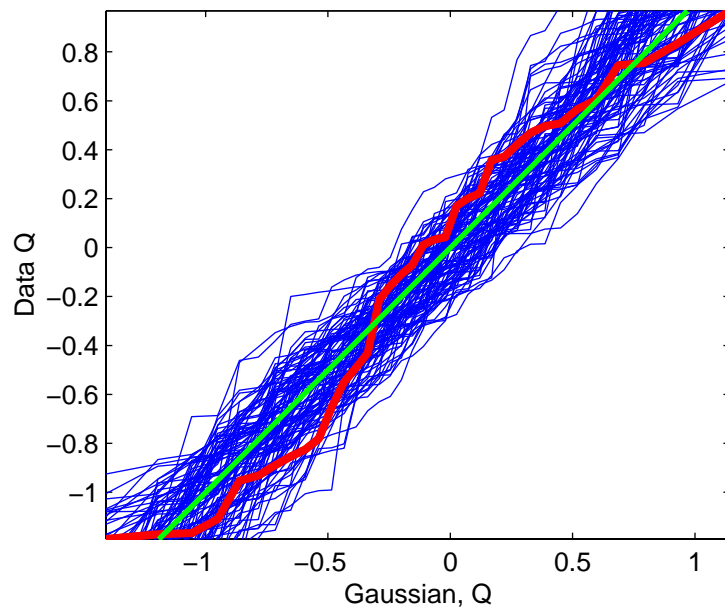
npc = 7 IC 3 Proj's, QQ
